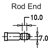
Rod End
